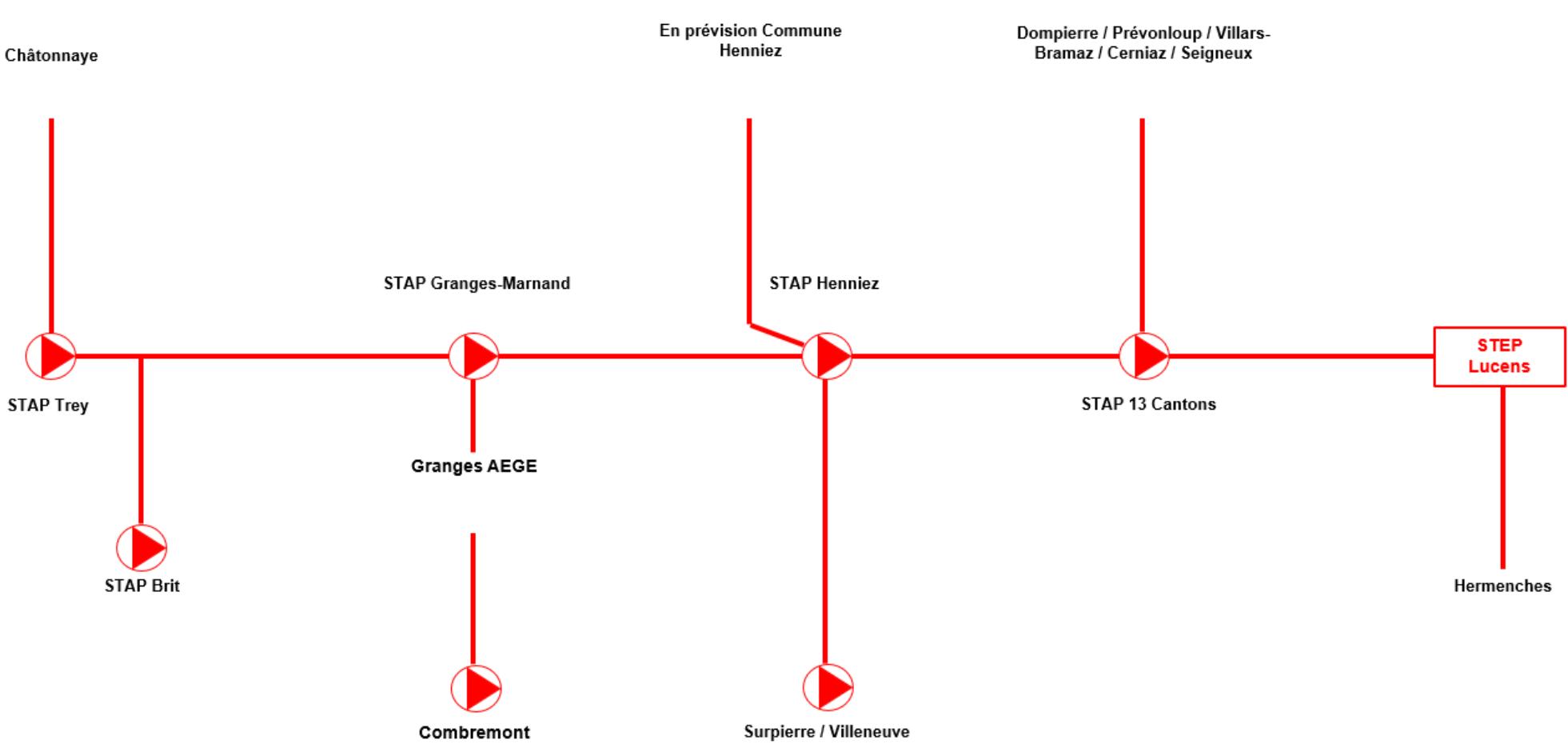
Schématique du réseau
