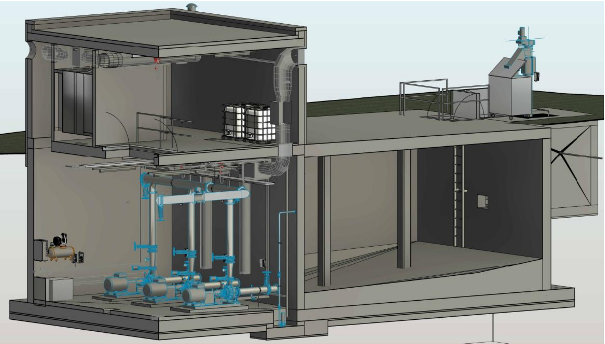
Modèle 3D STAP Treize Cantons
