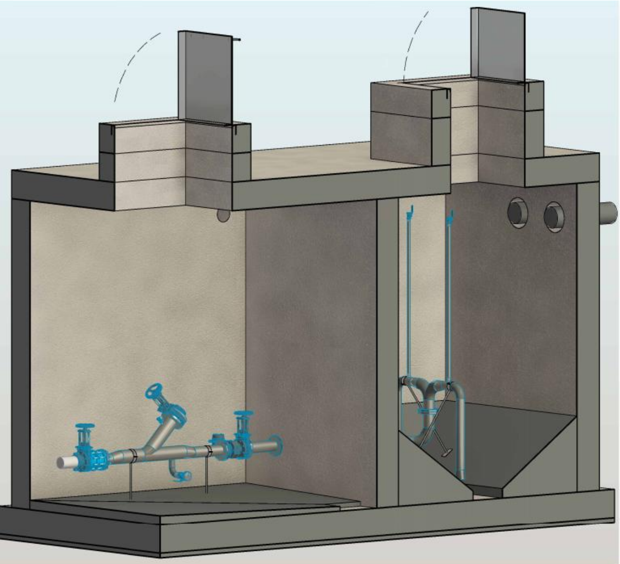
Modèle 3D puits de mise en charge d'Hermenches
