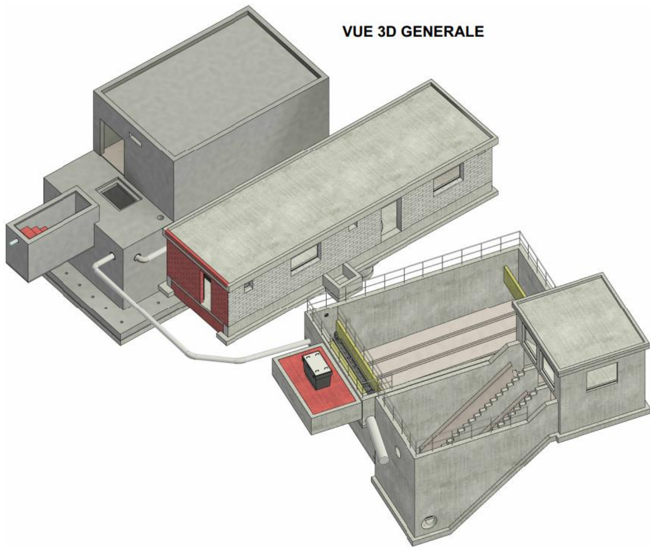
Modèle 3D transformation STEP de Granges-près-Marnand
