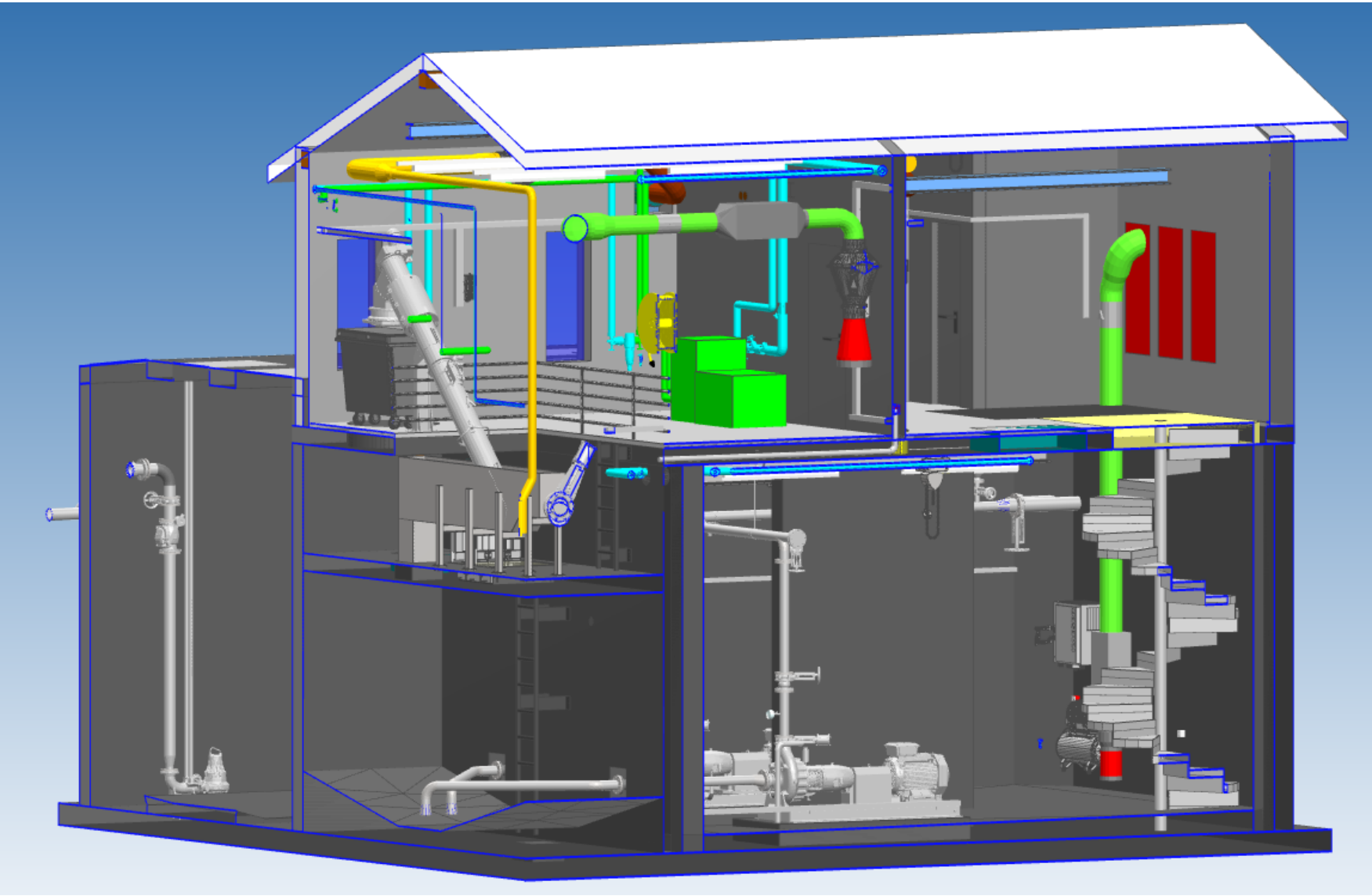
Modèle 3D STAP de Trey
